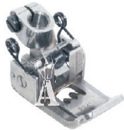
Piedino 3 aghi Presser foot (3 needles) cod. P0216 (3x5,6 mm) cod. P0217 (3x6,4 mm)
