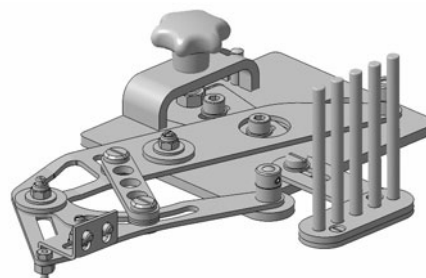
Bausatz für mitgehenden Einfasser Set for mobile binder
