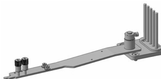
Trägerblech Carrier plate
