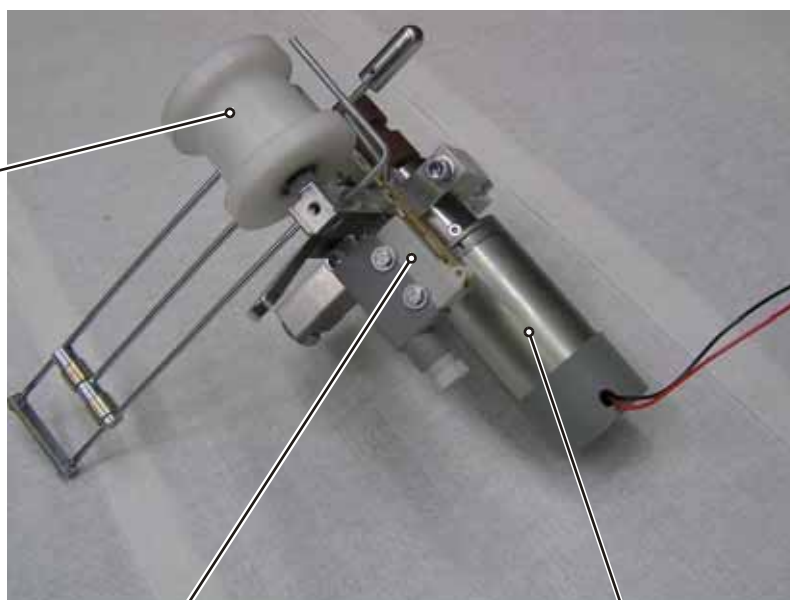
Mikroschalter micro switch 2000549.00
